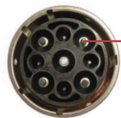
Varovalo za zaščito pred električnim udarom na vtiču JUICE CONNECTOR (m)
