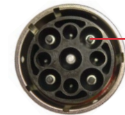
JUICE CONNECTOR -liittimen (m) sähköiskua estävä kosketussuoja
